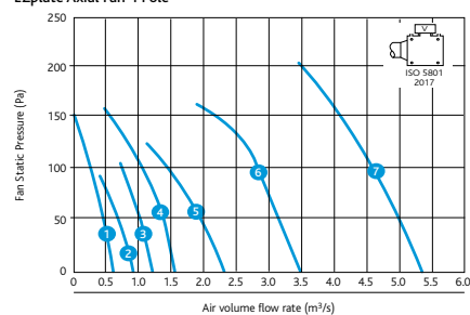
EZplate Axial Fan 6 Pole
