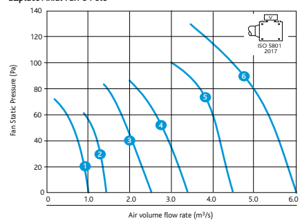
EZplate Axial Fan 8 Pole
