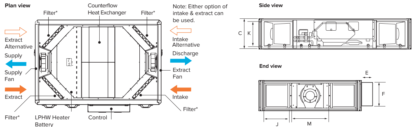
FAN CONFIGURATION
